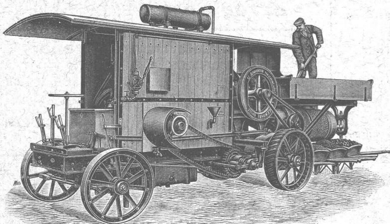
Concasseur automobile
