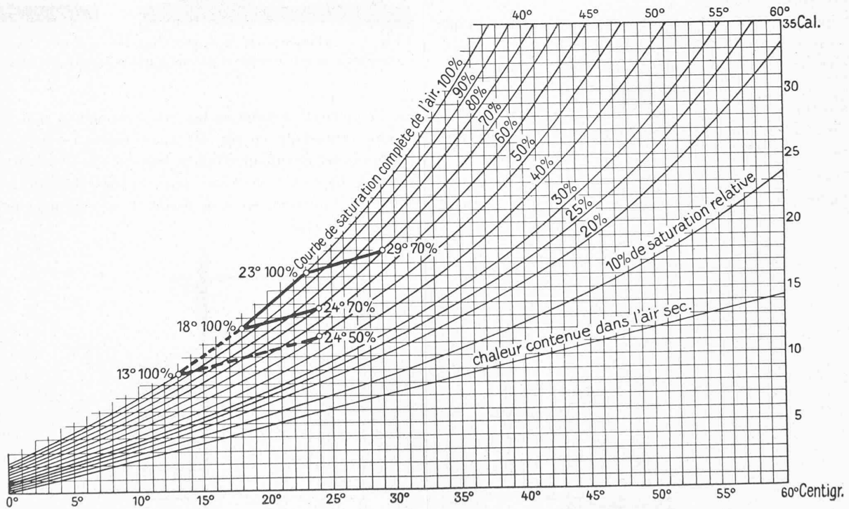
Fig. 13. — Représentation graphique du séchage de l'air en refroidissant et réchauffant de nouveau l'air à différentes températures.
