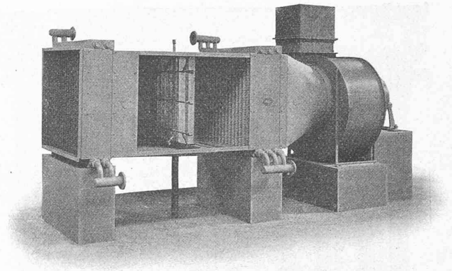
Fig. 10. — Appareil Sendric de chauffage, refroidissement et épuration de l'air, combiné avec un ventilateur Sulzer. Chauffage de 12000 m 3 d'air de -10° à +20° C.
