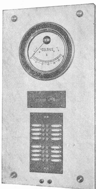
Fig. 2. Tableau de mesure pour thermomètres à résistance avec instrument indicateur et commutateurs à bouton.
