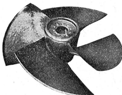
Roue à hélice d'une des 14 turbines de 2500 ch. chacune de l'usine de Wynau sur l'Aar.
