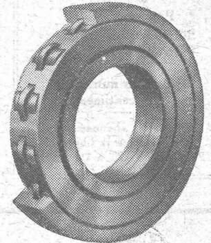
Roulements Jæger à rouleaux à collet pour efforts radiaux et axiaux.
