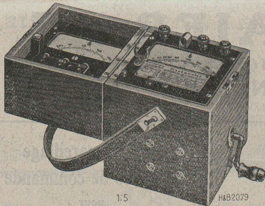
1:5 H&B2079 Mesureur d'isolement avec voltmètre.
