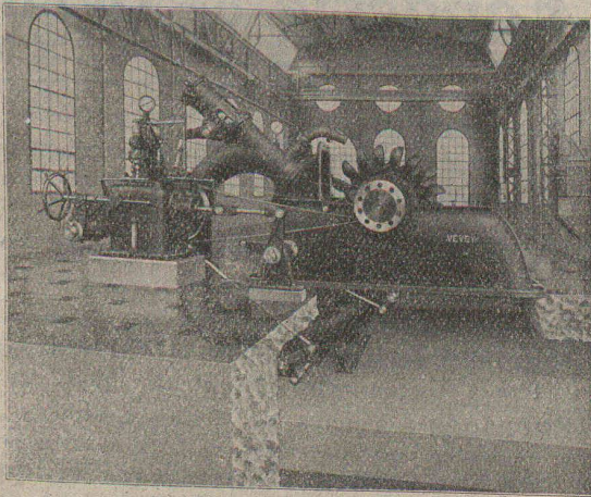
Une des turbines de l'usine de la Peuffaire (Cie vaudoise des Forces de Joux & de l'Orbe). — Puissance: 5000 ch. — Chute: 390 m. — Vitesse: 750 t: min.
