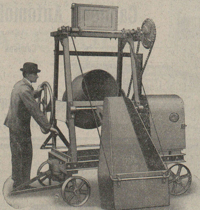
Notre nouvelle bétonnière basculante ainsi que concasseurs en diverses exécutions, pour rendement de 10 à 400 m 3 par jour.
