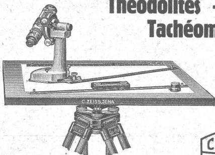
Alidade tachygraphe
