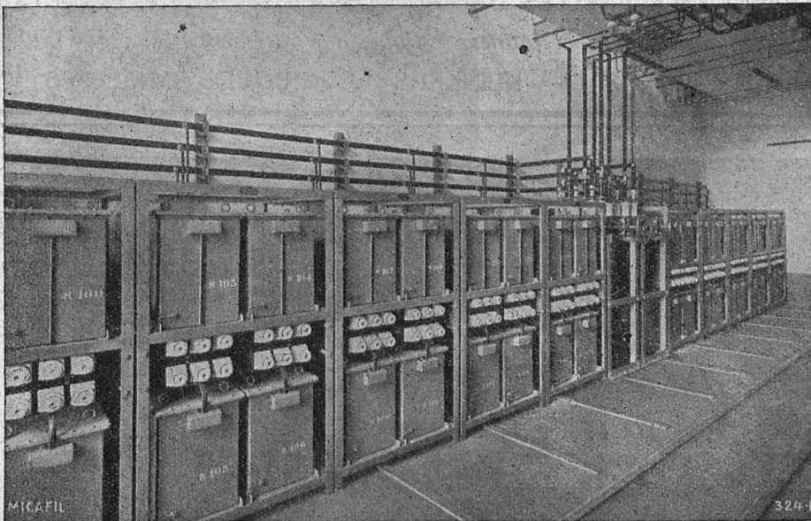
Batterie de condensateurs MICAFILE à la sous-station de Gruningen (Canton de Zurich) Puissance réactive : 1100 kVA, tension : 600 volts, 50 pér.
