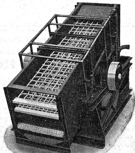
Le laveur vibratoire remarquable par son triage précis et son encombrement réduit.
