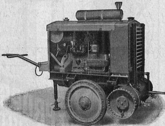
Moteur-compresseur léger type LZ. 20 pour l'actionnement d'un gros marteau perforateur ou d'un brise-béton. Léger, souple, économique.
