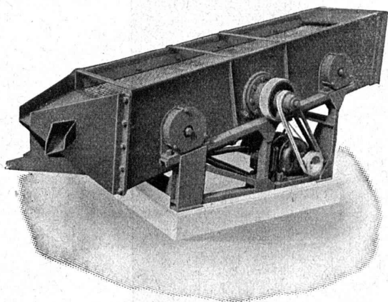
Tamis vibratoire nouveau modèle, fonctionnement sûr, trriage impeccable.
