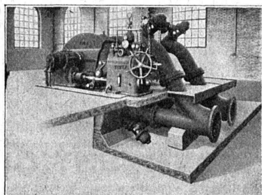
Turbine "Pelton", à 4 injecteurs. (Usine de Sernf-Niedererbach.)
