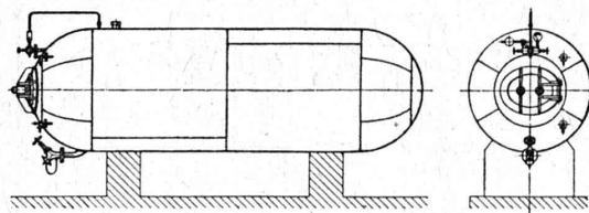
Tank à mûts, en acier inoxydable. Pression d'acide carbonique : 7 atm.
