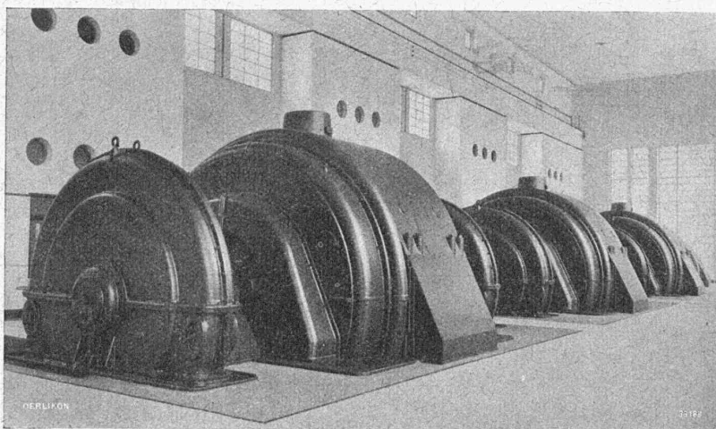
Centrale La Dixence de la E. O. S., Lausanne. 5 alternateurs Oerlikon chacun de 37 500 KVA, 13 kV, 50 pér., 500 tours min. et un alternateur Oerlikon de 9000 KVA.
