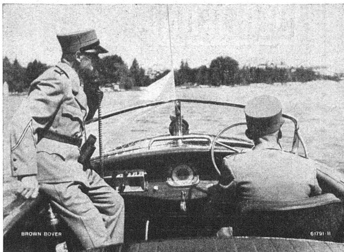
Ce canot patrouilleur de la police municipale de Zurich est équipé d'un émetteur à ondes ultra-courtes et d'un récepteur à ondes courtes. De ce fait le chef de patrouille peut se mettre à tout moment en communication dans les deux sens avec le poste de commandement.
