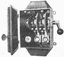
500 V. 25 A.
