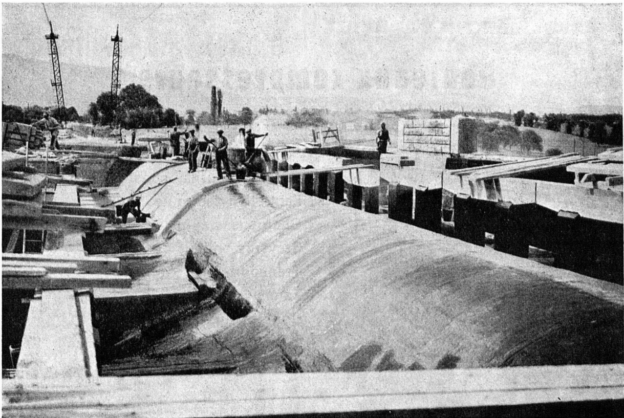
Pont Butin, Genève. — Etanchéité des voûtes exécutée en asphalte souple «Système Hirschy», effectuée il y a 25 ans.
