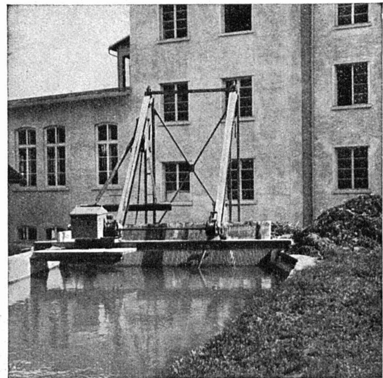
Appareils dégrilleurs
