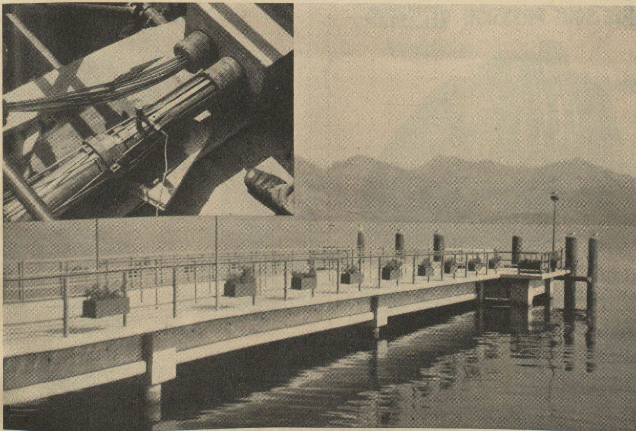
Débarcadère de Nyon reconstruit en 1947 en béton précontraint — Exécutant : ENTREPRISE LOSINGER & Cie S. A., Lausanne A gauche en haut : Deux ancrages de câbles et le vérin de précontrainte (voir page 12 du présent numéro).
