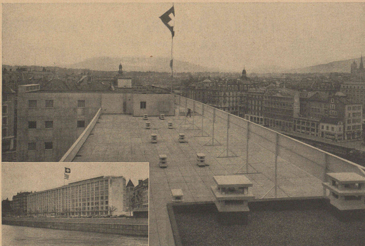
Hôtel du Rhône à Genève. — Etanchéité des toitures terrasses exécutées en asphalte souple « Système Hirschy » recouverte par dalles en ciment teinté.
