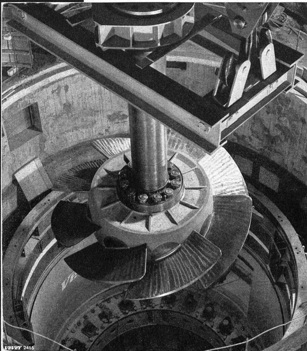
Usine de Lavey, roue Kaplan de 83 650 ch
