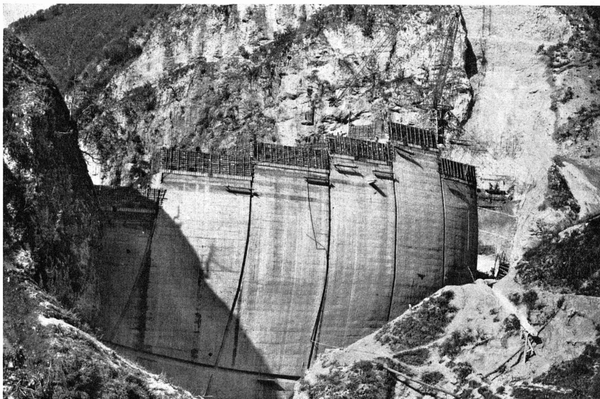
Barrage de Val Gallina, de la S.A.D.E., en béton au Plastiment.
