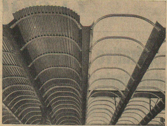
Avant-toit d'une entrée de gare. Voûtes en tonneau en bandes ondulées d'Aluman, profilées en arc et chéneaux autoportants en Anticorodal.
