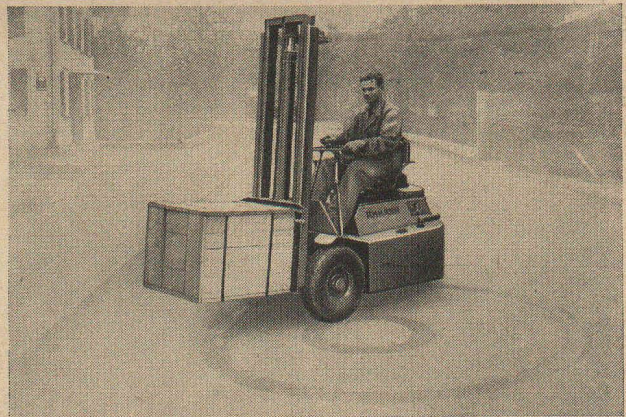
Chariot-élévateur
