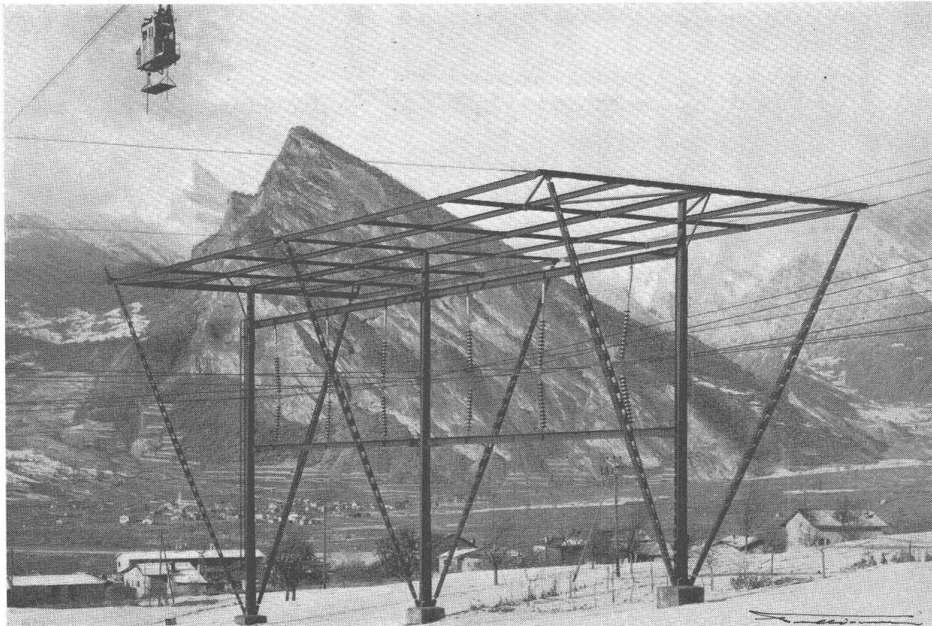
Portique porteur de la ligne H. T. Riddes-Sanetsch-Mühleberg avec plateforme de protection sous le téléphérique Riddes-Isérables.
