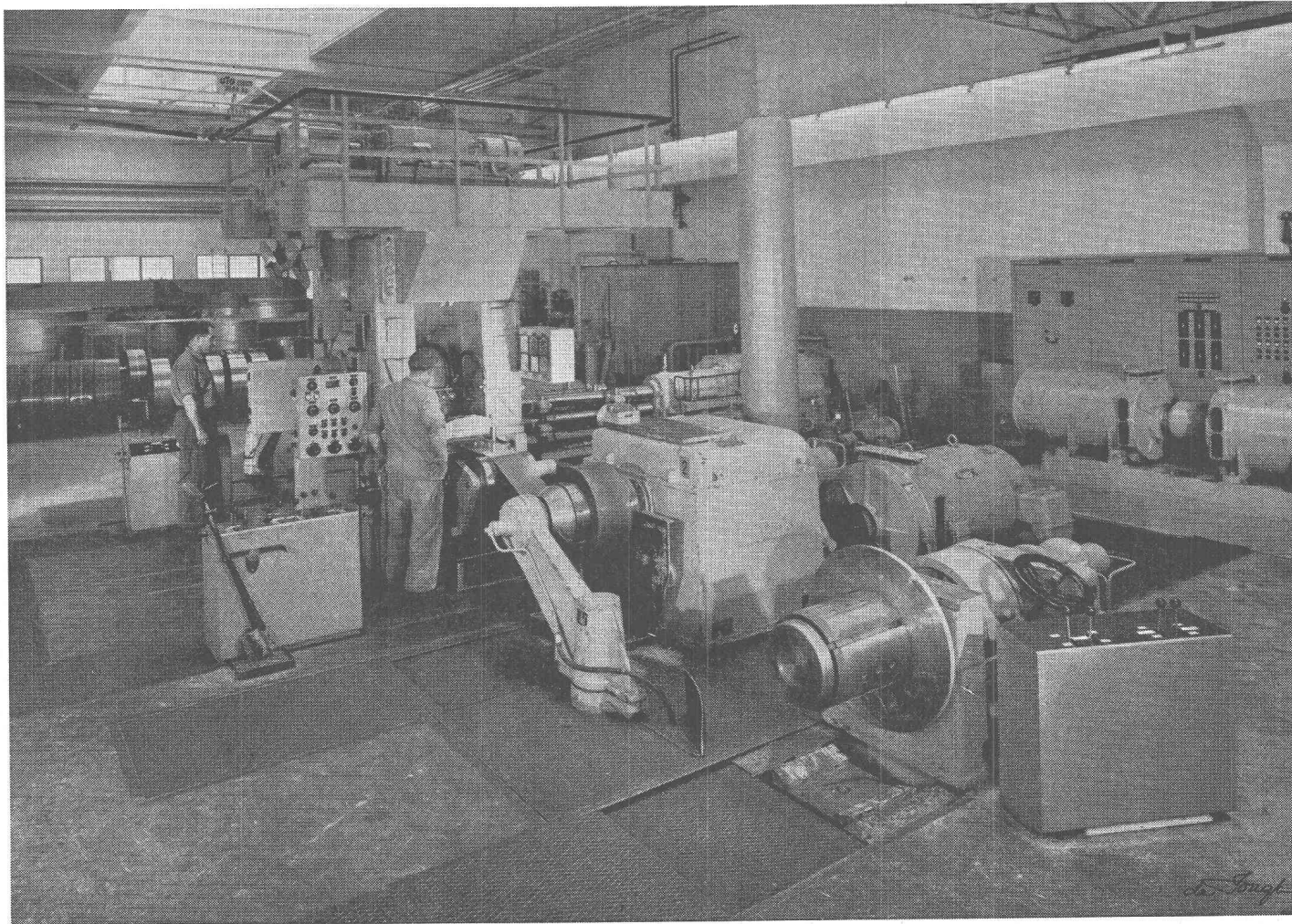
Laminoir quarto réversible à commande électronique pour le laminage de feuilards de fer. (Photo prise au Département de laminage de la S. A. des Câbleries et Tréfileries de Cossonay)
