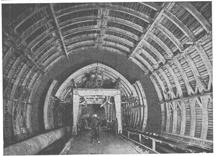
Coffrage télescopique pour le tunnel routier du Grand St-Bernard
