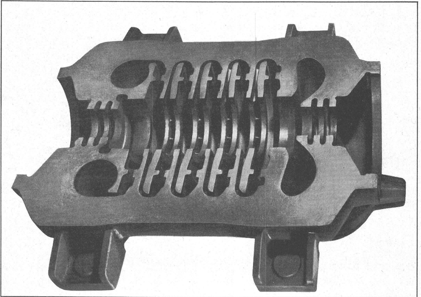
Partie inférieure d'un corps de turbosoufflante, en fonte sphérolitique perlitique SG 58; poids unitaire 650 kg
