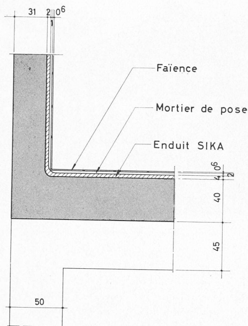
Fig. 3. — Etanchéité du bassin olympique.
