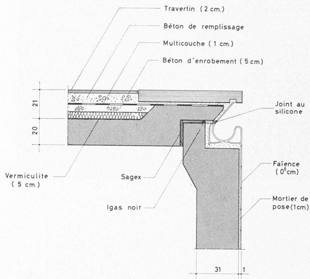
Fig. 4. — Joint horizontal de dilatation entre le bassin olympique et la dalle du niveau baigneurs.
