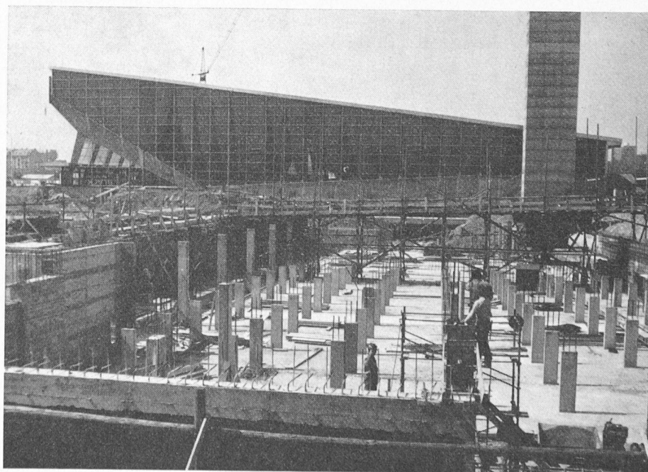
Fig. 5. — Infrastructure du bassin olympique.
