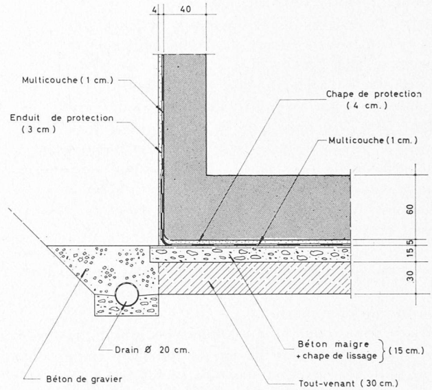
Fig. 2. — Coupe détaillée du sous-radier et du radier.
