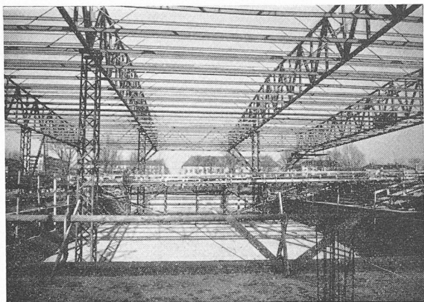
Fig. 6. — Structure métallique constituant le grand lanterneau.
