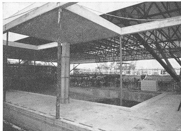
Fig. 7. — Champignon en béton armé du pourtour du grand lanterneau.
