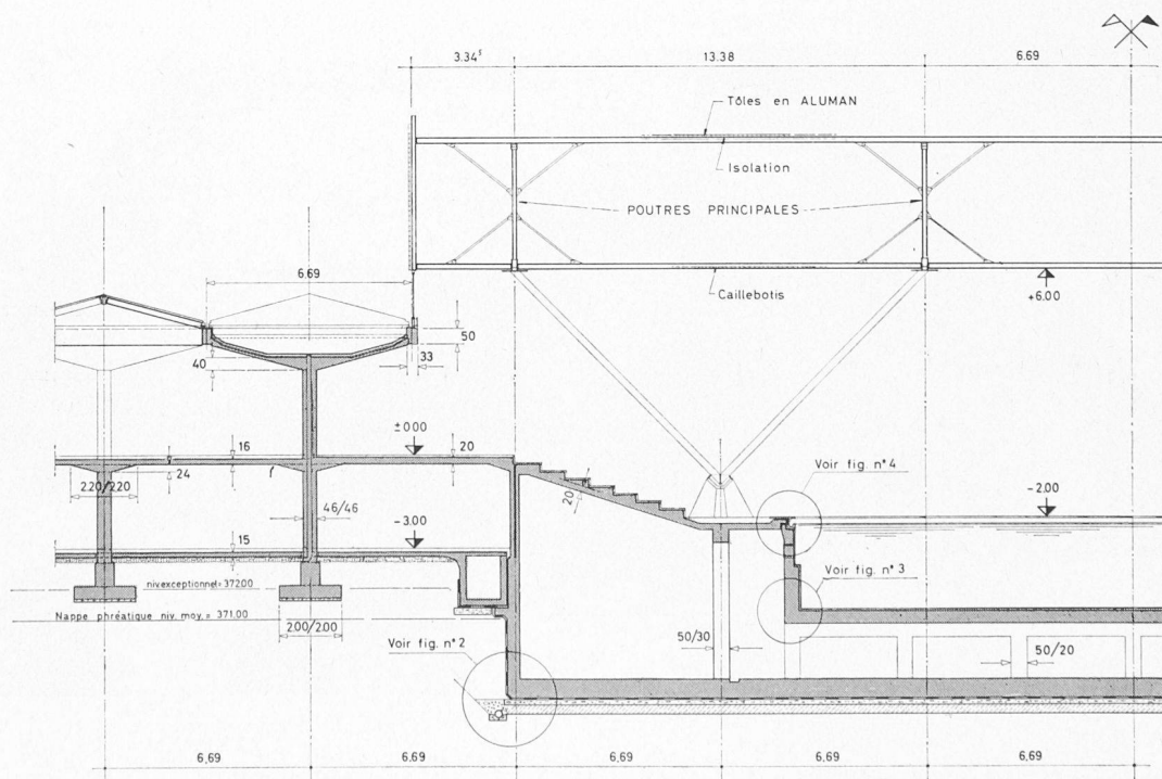
Fig. 1. — Coupe générale montrant à gauche une partie de la zone des vestiaires et de l'administration et à droite une partie de la zone de la piscine.
