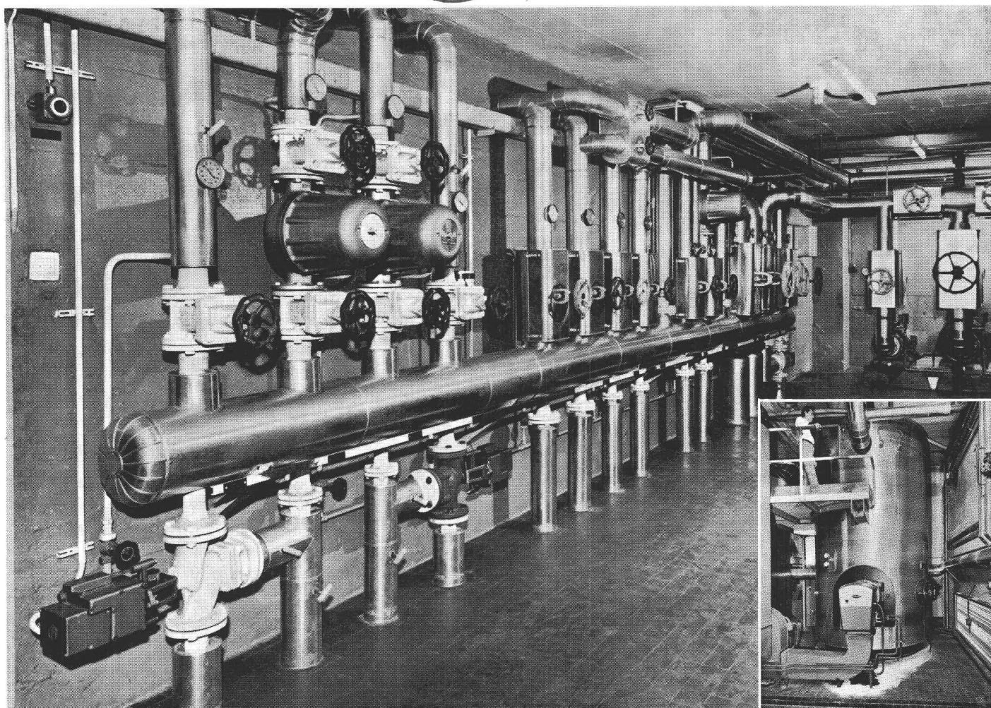
Sous-station "Usine II" et installation de la nouvelle chaudière Sunrod d'une puissance de 5.000.000 kcal/h. 130°C.
