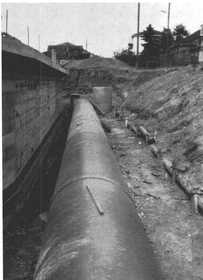
Commune de Bussigny près Lausanne Collecteur d'eaux de surface \varnothing 125 cm
