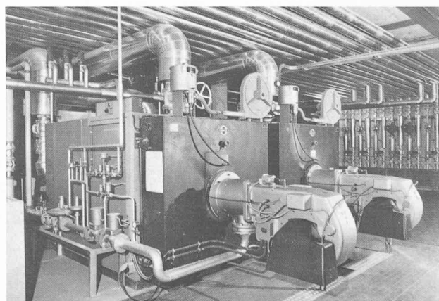
Fig. 17. — La chaufferie avec au premier plan l'alimentation en gaz.
