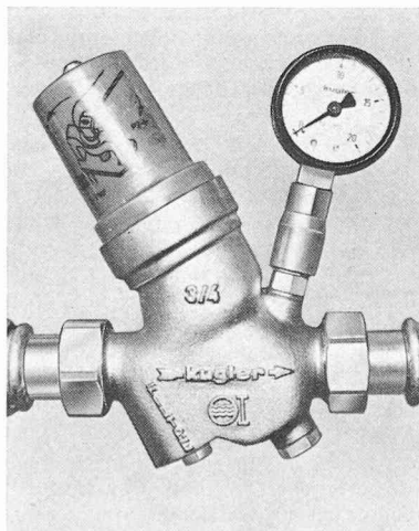
Réducteur n° 7416 avec pression indépendante de la pression primaire grâce au compensateur incorporé.
