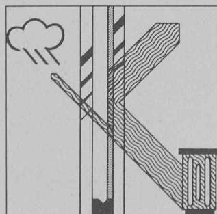
Fig. 1. — Principe fonctionnel du vitrage Thermoplus: Le vitrage permet à la lumière naturelle de pénétrer dans le local, mais empêche la chaleur du chauffage de s'échapper, et tout cela grâce à un vitrage isolant composé de deux feuilles de verre.
