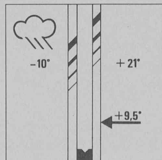
Fig. 2. — Avec un vitrage isolant normal présentant un coefficient k de 3,0 W/m 2 K, la température ambiante baisse considérablement à la surface du vitrage; c'est la raison pour laquelle il est désagréable de s'asseoir ou de travailler à proximité de la fenêtre durant l'hiver.
