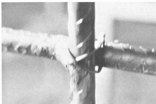
Fig. 12. — Liaison d'armatures par soudure.
