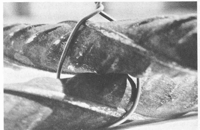
Fig. 11. — Liaison d'armatures par le système de ligature traditionnelle.
