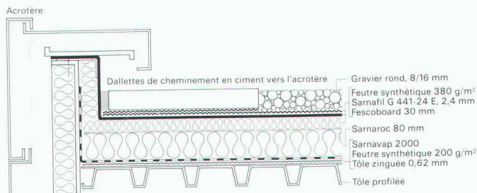
Construction de couches d'un toit plat Sarnafil sur des tôles profilées.
