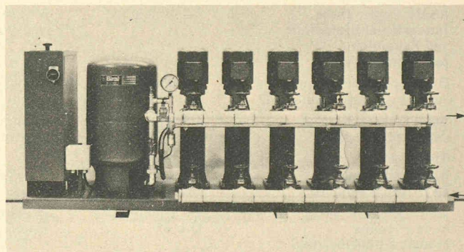
Surpresseur automatique Biral DWA-P commandé par microprocesseur pour l'amortissement des coups de bélier dans les réseaux fortement sollicités.
