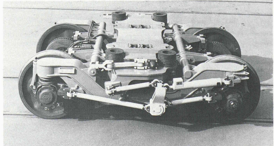
Fig. 2. - Conception modulaire. De haut en bas: - bogie SIG équipé du système Neiko - bogie SIG équipé du système Navigator - bogie SIG équipé de la combinaison Neiko-Navigator.
