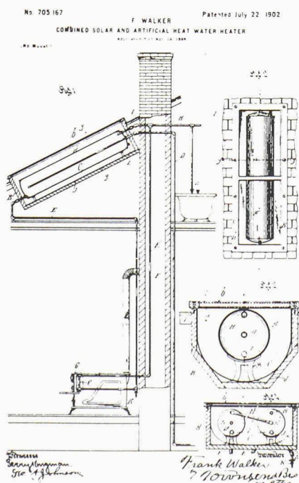
Fig. 2. – Copie du brevet de chauffe-eau solaire déposé par Frank Walker en 1902 à Los Angeles.
