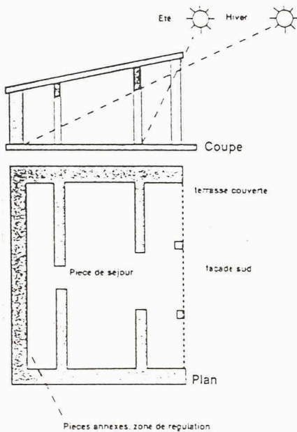
Fig. 1. – Conception d'une maison solaire selon Socrate (environ 400 ans avant J.-C.).
