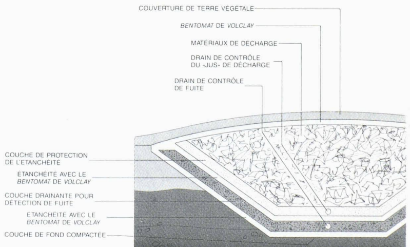
Etanchéité d'une décharge: schéma de principe
