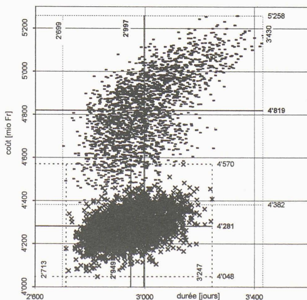
Fig. 2.- Diagramme temps-coûts du génie civil pour le tunnel de base du St-Gothard. Le nuage du bas (x) correspond à la variante actuellement confirmée quant à la composition de la zone de Piora au niveau du tunnel.
