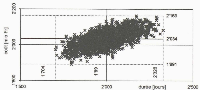
Fig. 1.- Diagramme temps-coûts du génie civil pour le tunnel de base du Lötschberg (1 an correspond à 320 jours de travail).
