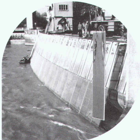
Grille de la prise d'eau du barrage de Lavey - VD Conduite forcée de Lucendro - TI
