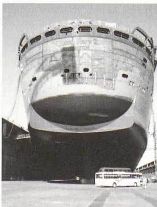
Chantier Queen Mary 2 (Document Cunard Line)
