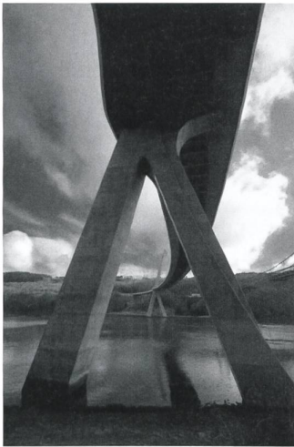
Le pont de Térénez (Finistère) vu depuis la rive gauche de l'Aulne. A droite, on distingue l'ancien ouvrage en cours de déconstruction. (Photo Paul Fulbert - Agence LAVIGNE CHERON)
