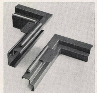
norm Türzargen
