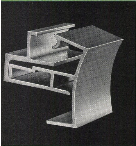
Gliasa-Schauenster-Rahmen-Konstruktion
