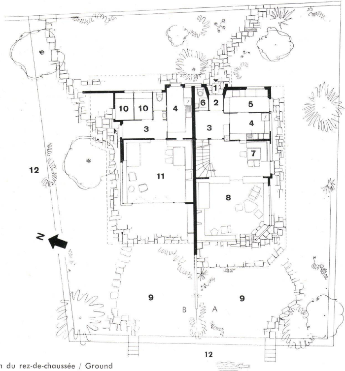
Grundriß Erdgeschoß / Plan du rez-de-chaussée / Ground floor plan 1:250
