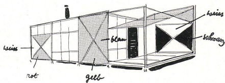
Perspektivskizze mit Farbangaben. Dessin perspectif et indications des couleurs. Perspective sketch with colour indications.
